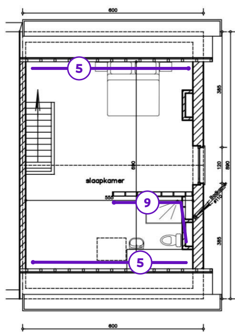
dakverdieping bestaand te regulariseren
