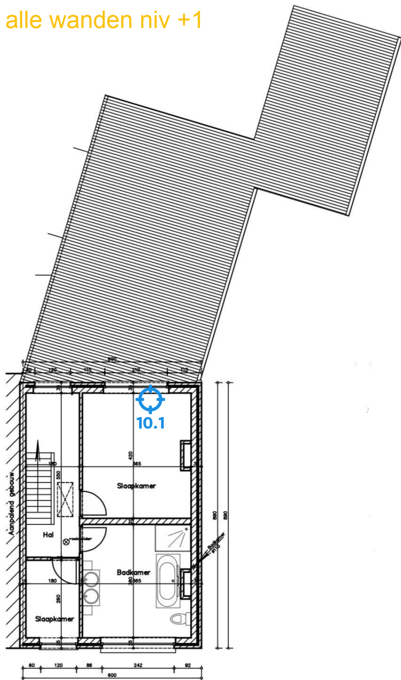
1° verdieping bestaand te regulariseren
